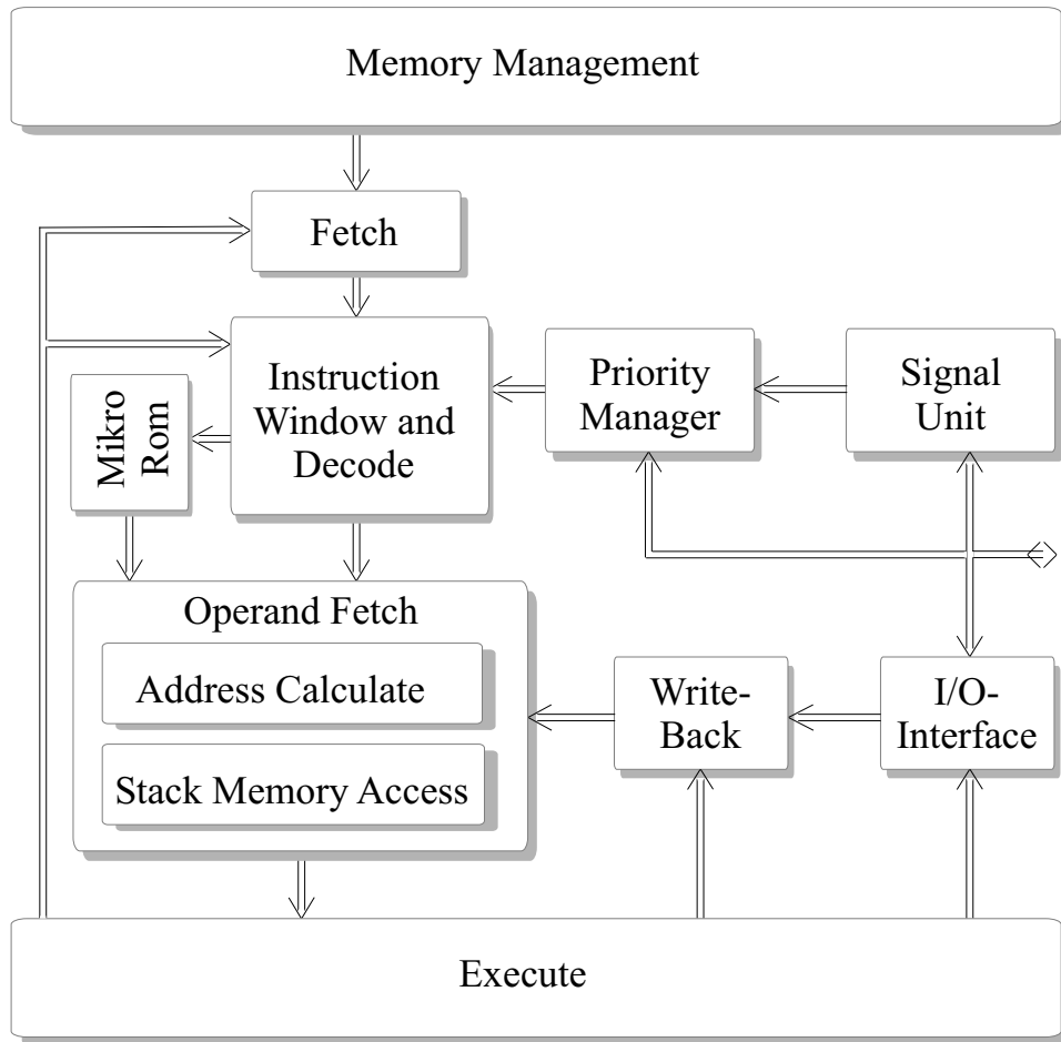
Abbildung 1: Die Komodo-Pipeline
